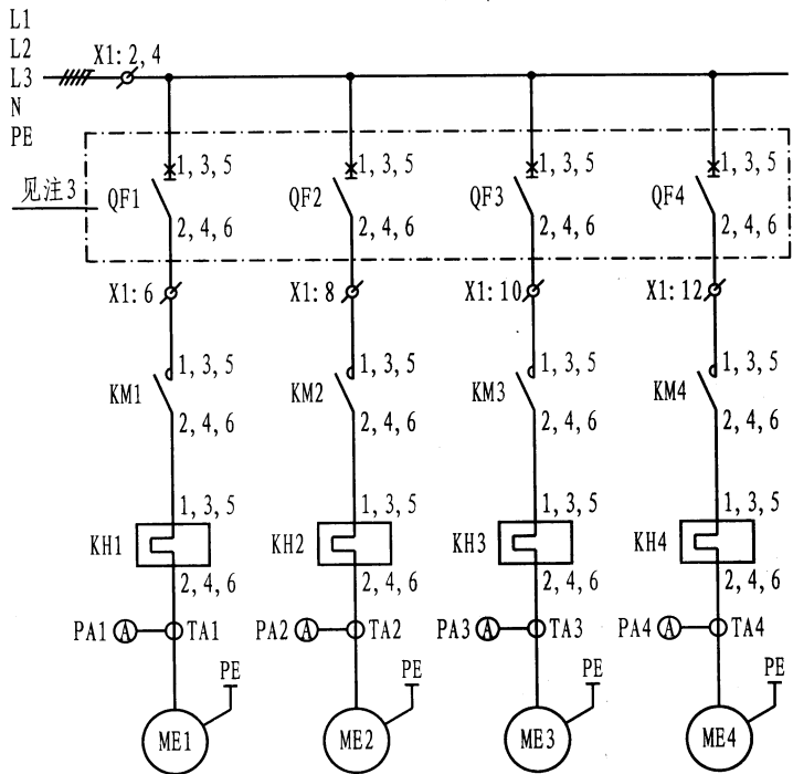
主回路
