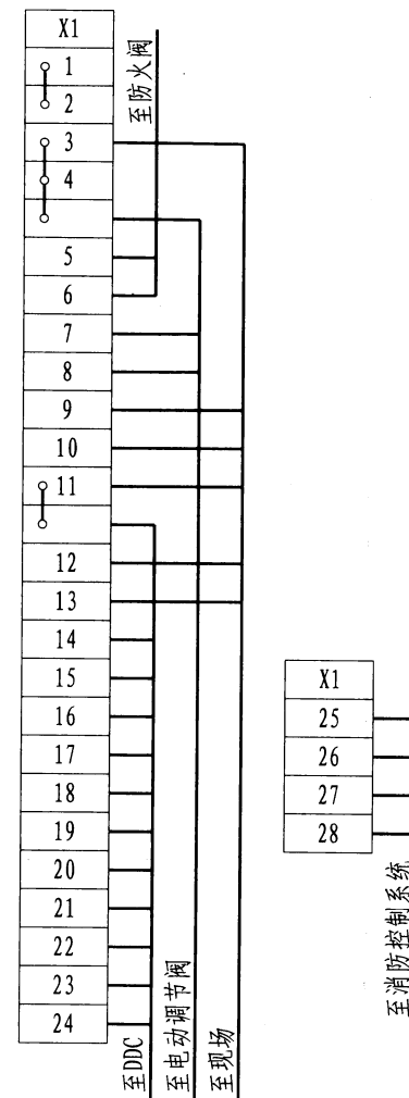
外部接线图
