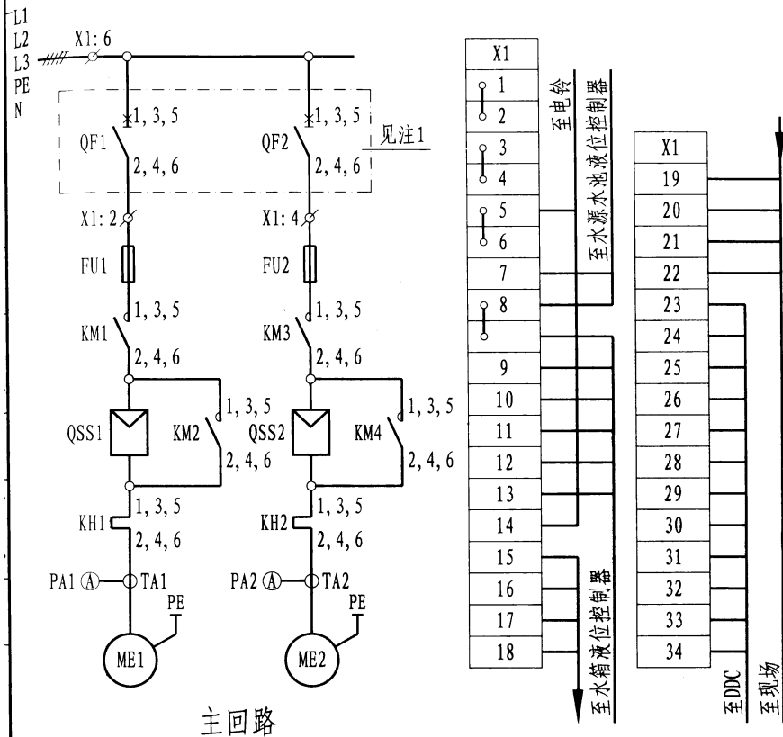
外部接线图
