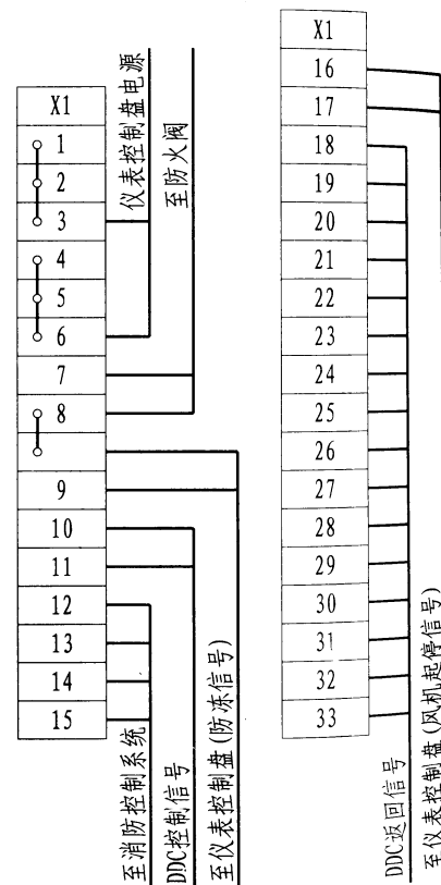
外部接线图
