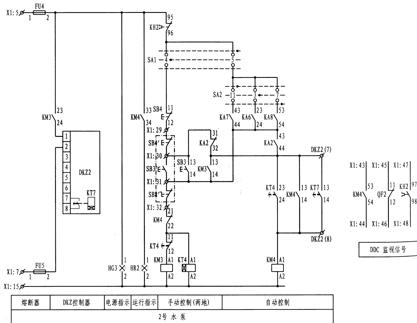
控制原理图
