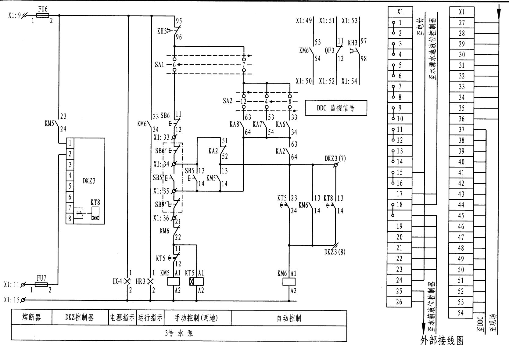
控制原理图
