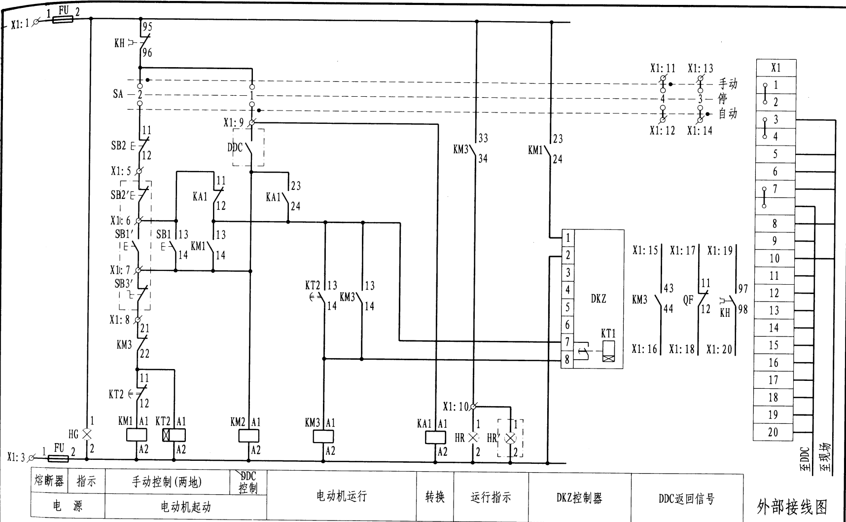
控制原理图
