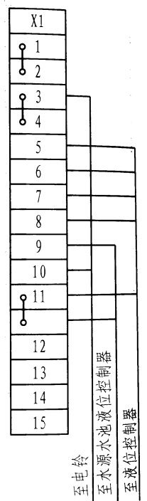
外部接线图
