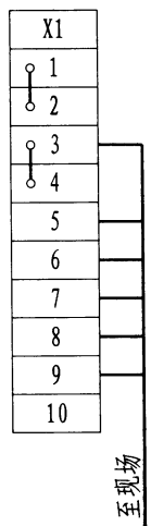
外部接线图
