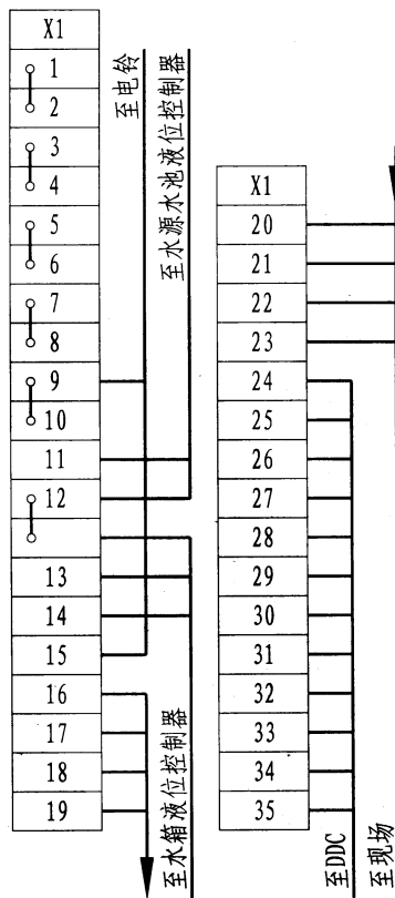
外部接线图
