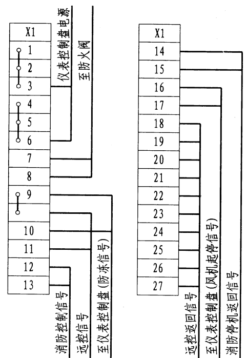
外部接线图
