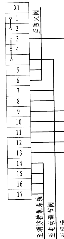
外部接线图
