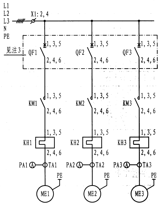
主回路
