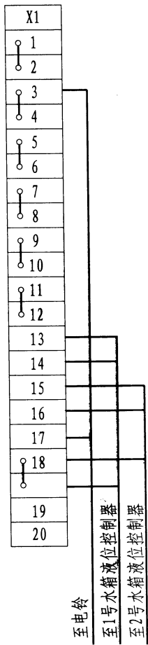
两组水泵可编程序控制器 控制装置电路图一
