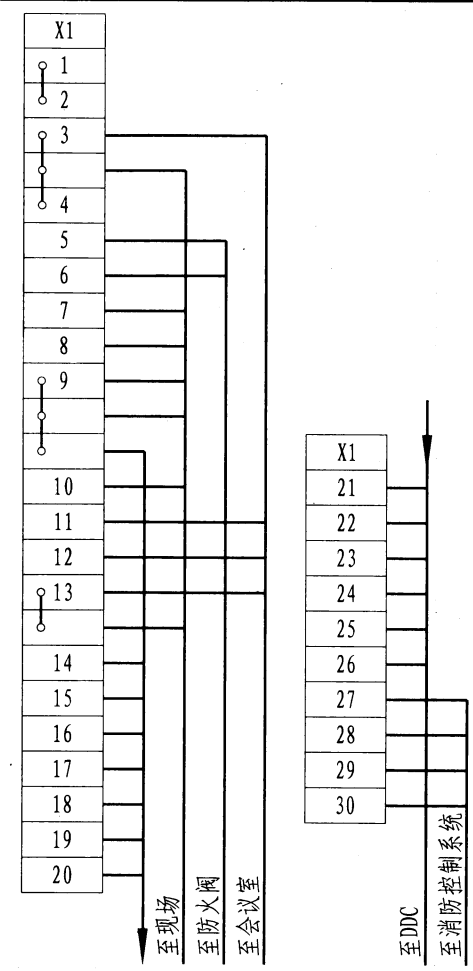
外部接线图
