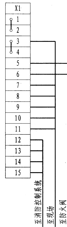
外部接线图
