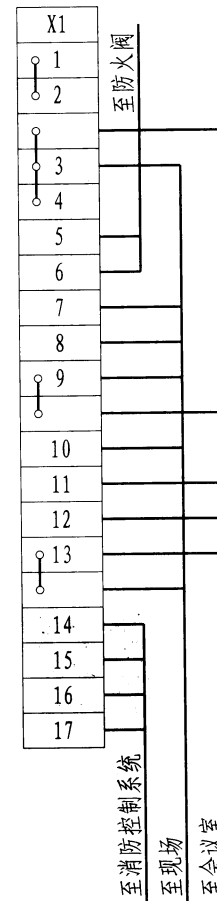
外部接线图
