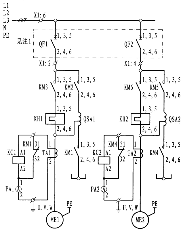
主回路
