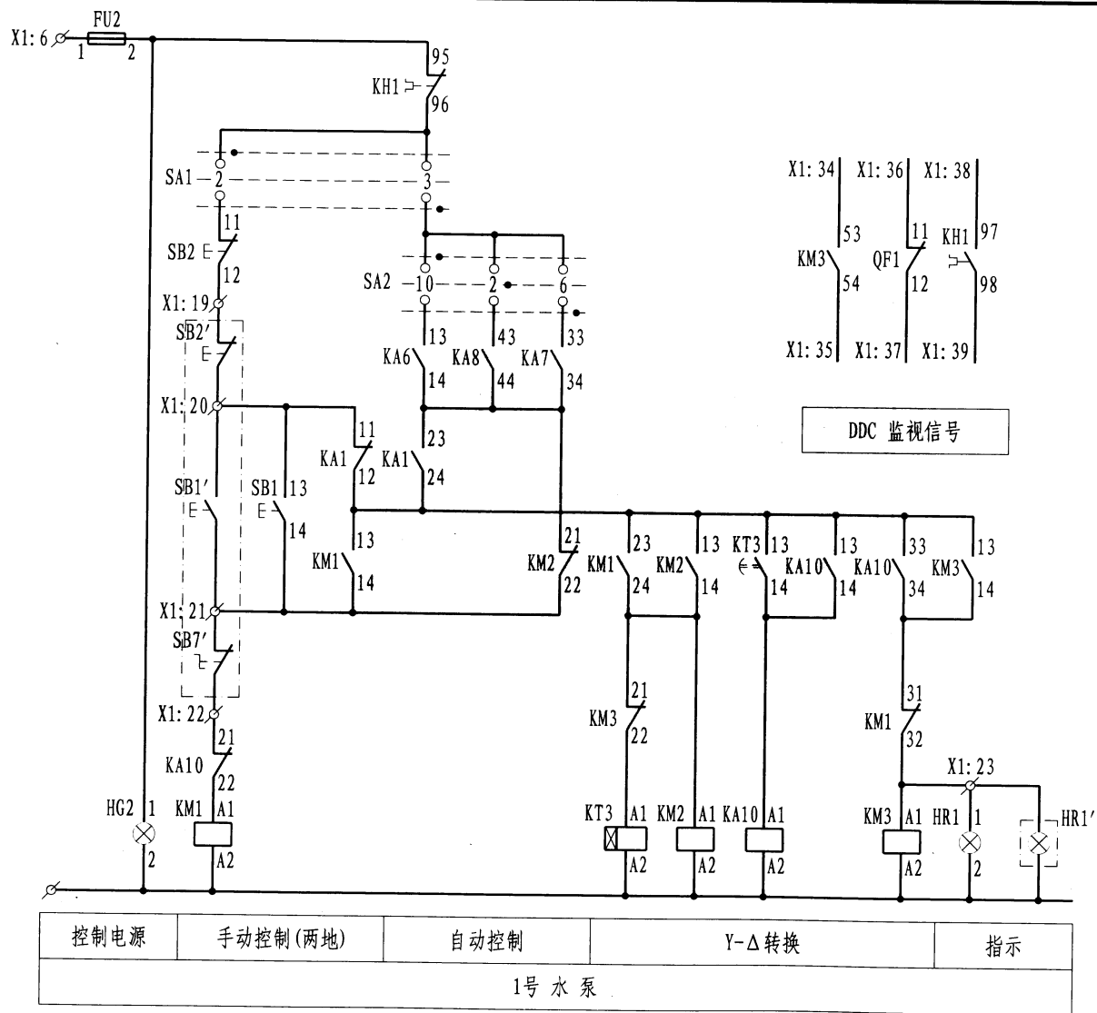
控制原理图
