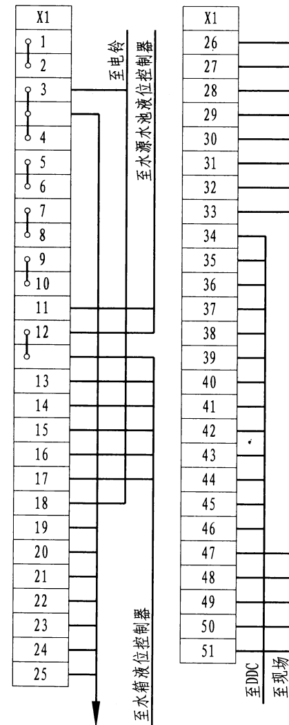
外部接线图
