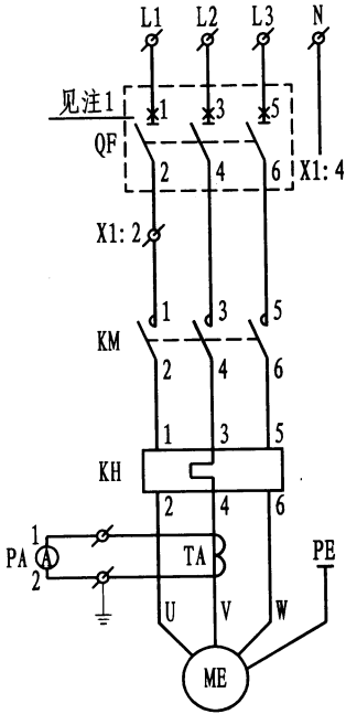
主回路
