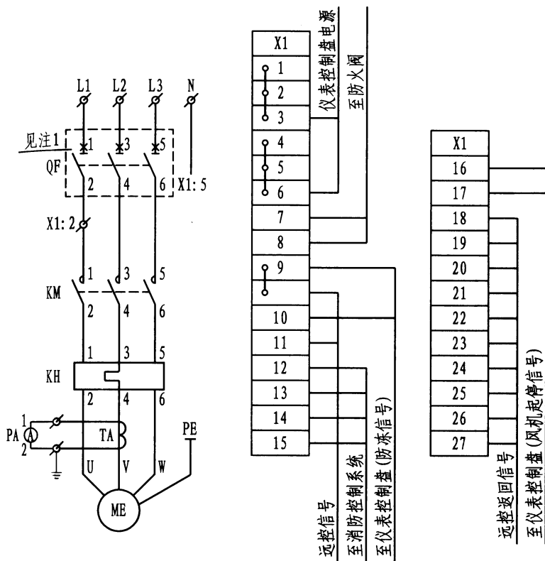
主回路
