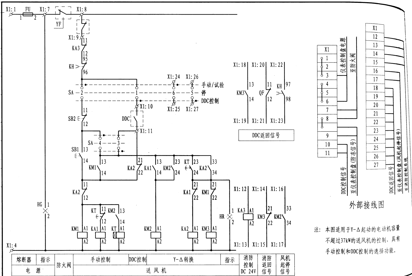
控制原理图
