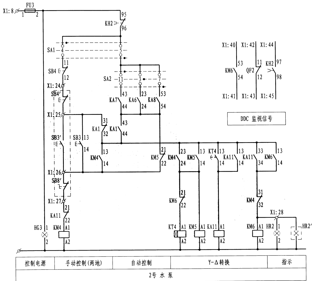
控制原理图
