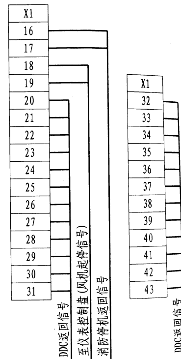
外部接线图
