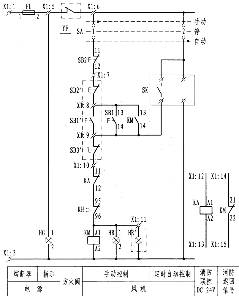
控制原理图
