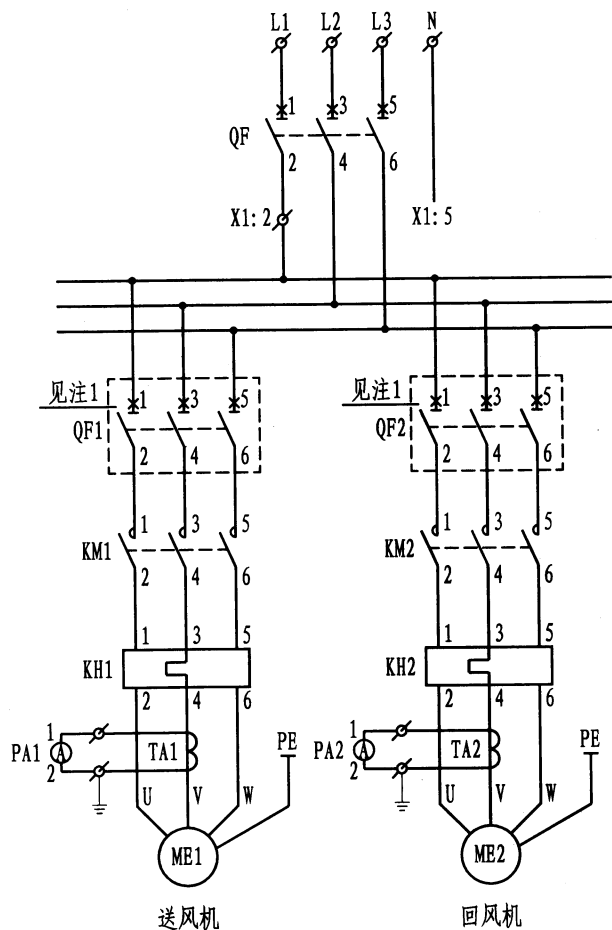
主回路
