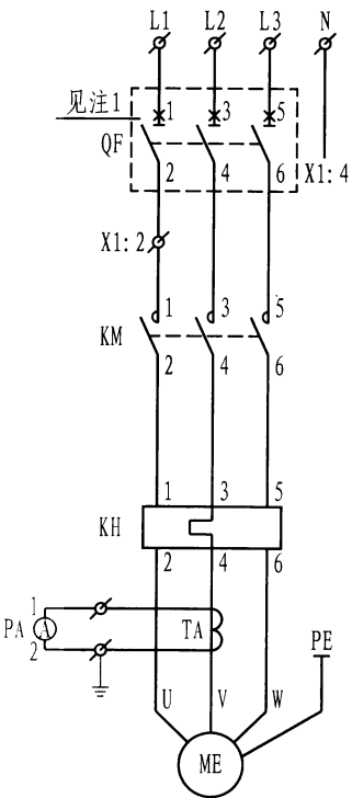
主回路
