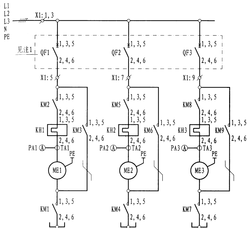
主回路
