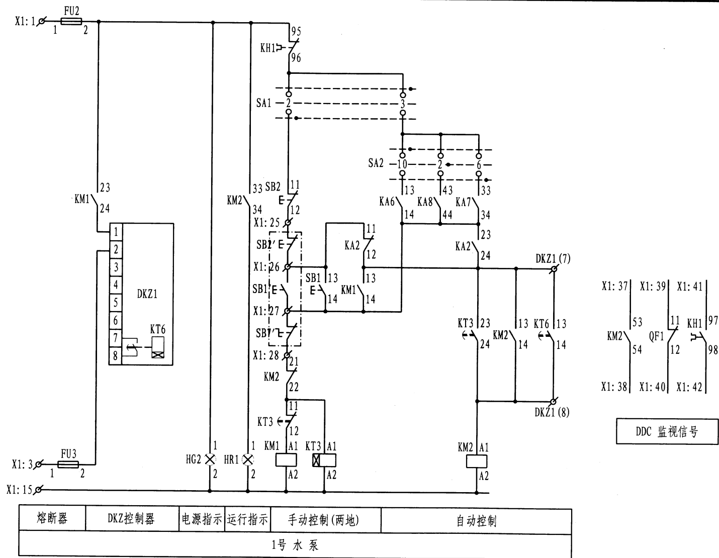
控制原理图
