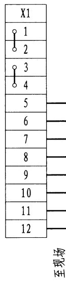
外部接线图
